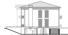
Elevation 04
